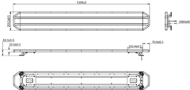
Afmetingen SL5-1359A
