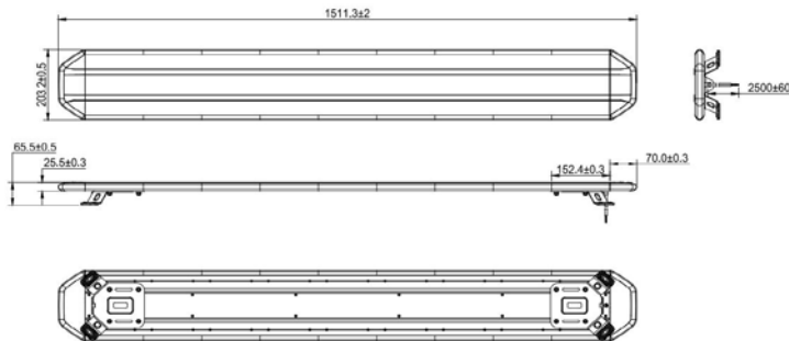
Afmetingen SL5-1511A
