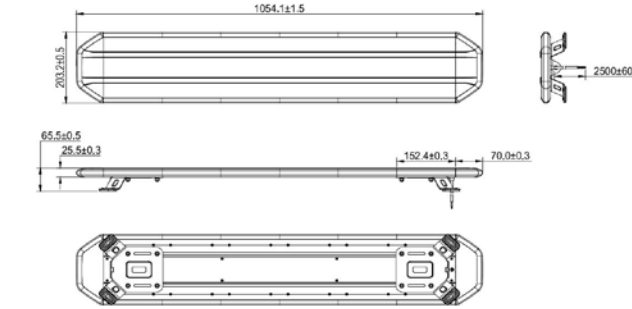
Afmetingen SL5-1054A
