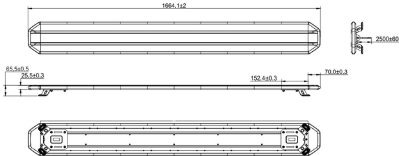
Afmetingen SL5-1664A
