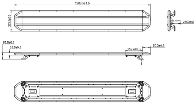
Afmetingen SL5-1206A
