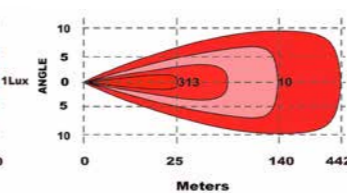
Lichtbeeld Skytrack 2
