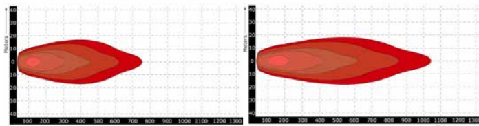
Lichtbeeld TRSW12278-1D
