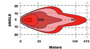
Lichtbeeld Geminus 1
