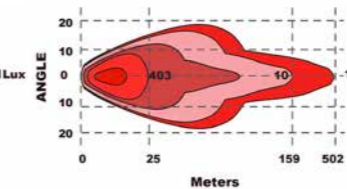
Lichtbeeld Geminus 2
