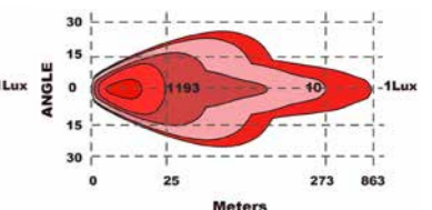
Lichtbeeld Geminus 4
