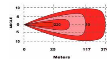
Lichtbeeld Shadow 1
