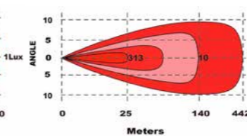
Lichtbeeld Shadow 2
