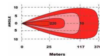
Lichtbeeld Skytrack 1
