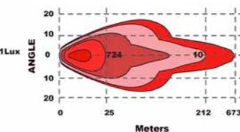
Lichtbeeld Geminus 3
